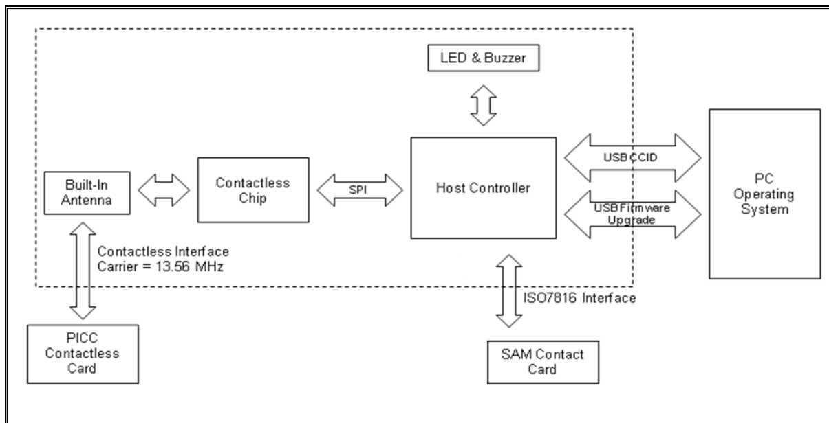
图1: ACR1552U 读写器功能框图
