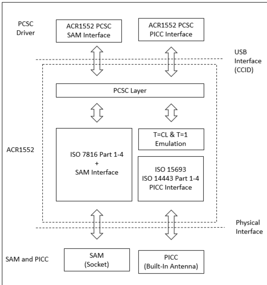
图2: ACR1552U 的结构
