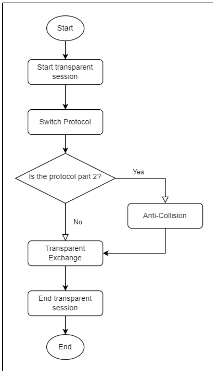
图5：ACR1552U 透明会话流程图
