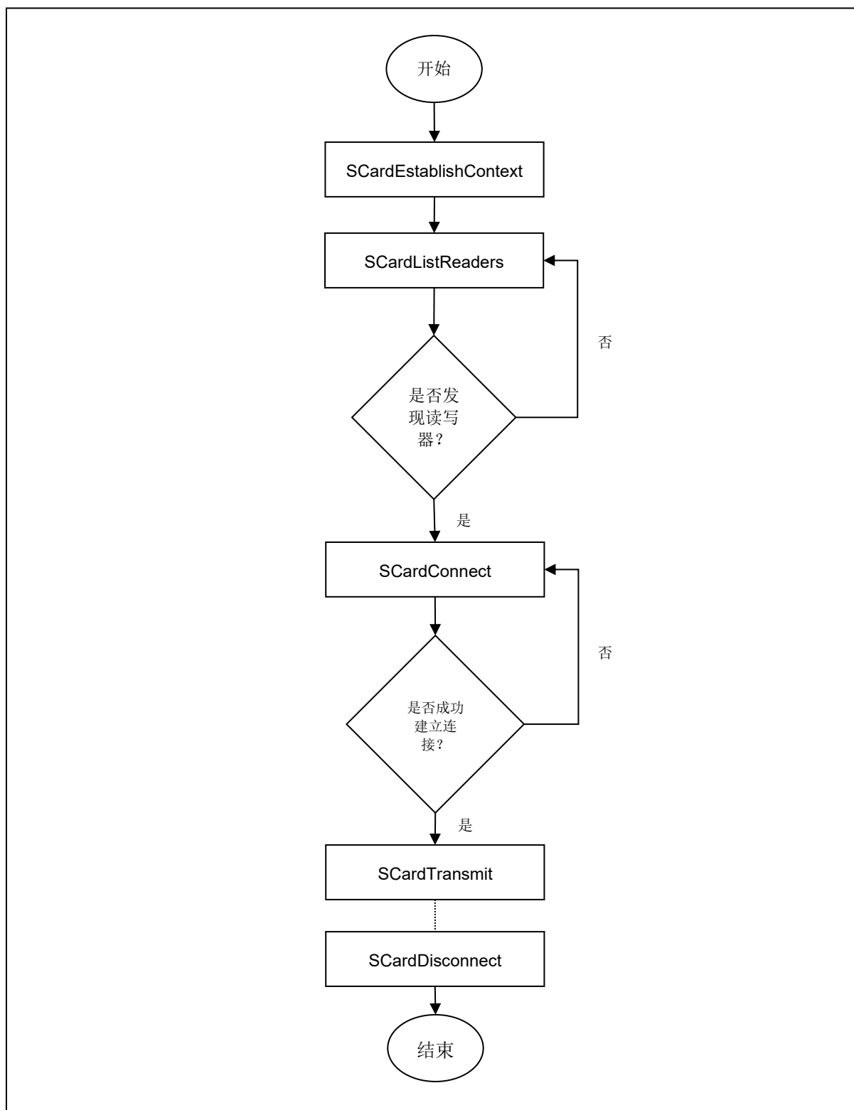
图3: ACR1552U APDU 流程图
