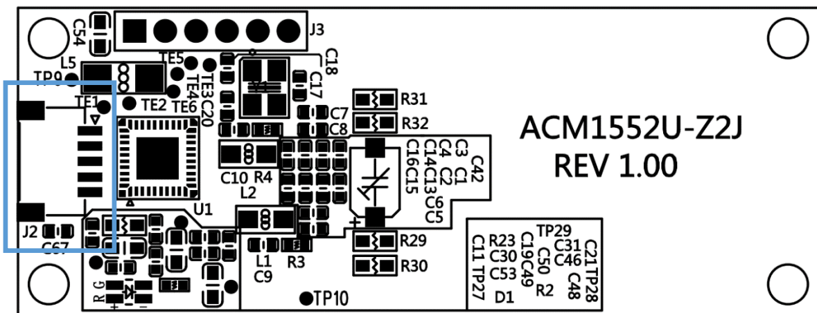
图 1: ACM152U-Z 的 USB 配置
