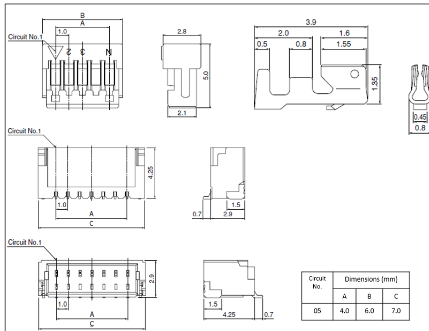
图 3: ACM1552U-Z 数据线连接器 (母头) 规格
