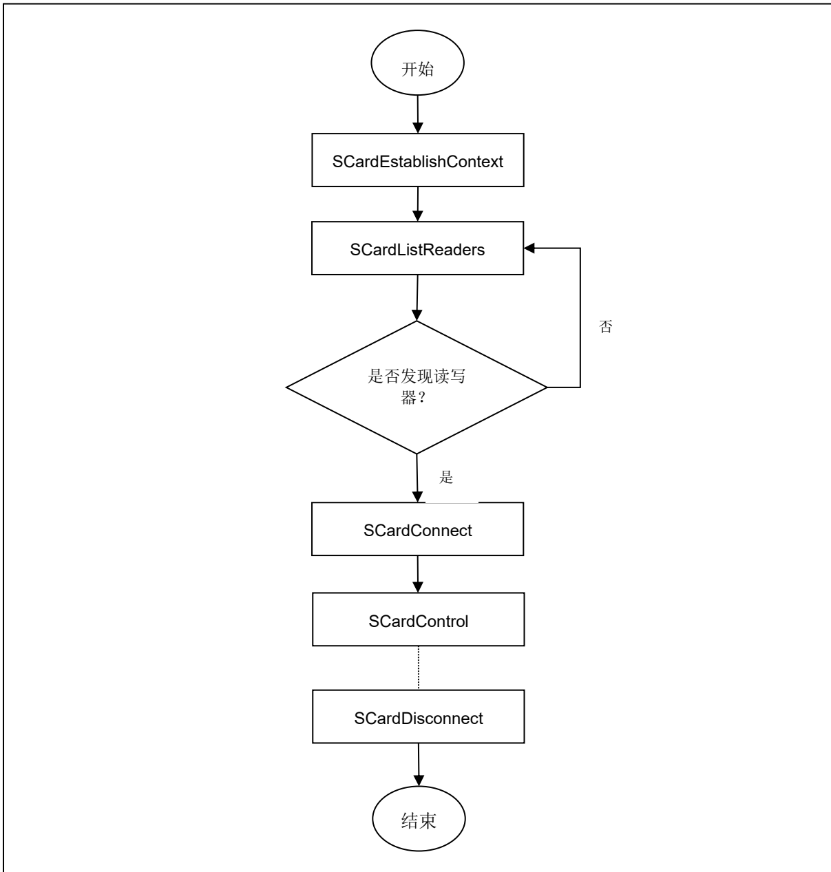
图 2: ACM1552D-C7 直接命令流程图
