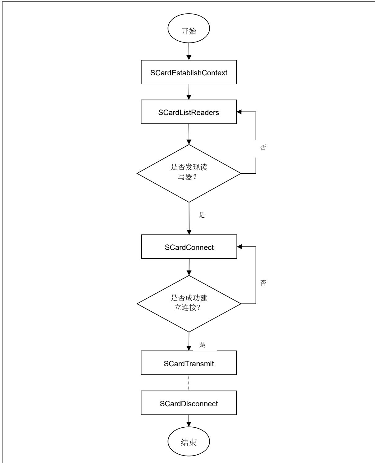
图 1: ACM1552D-C7 APDU 流程图
