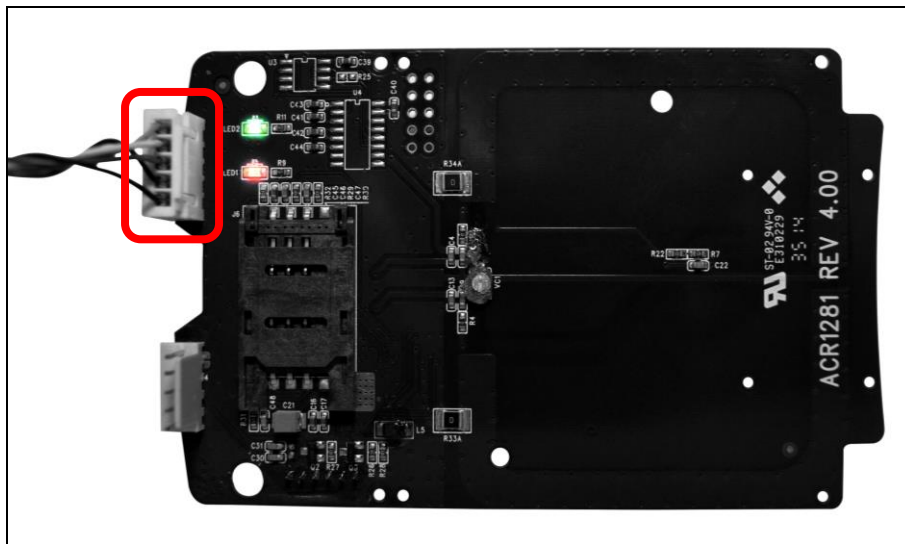
图4：ACM1281S-C（通过串口）
